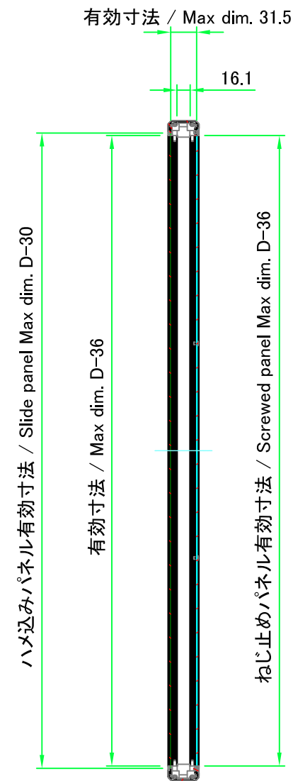
B-B ( 1 : 6.5 )
