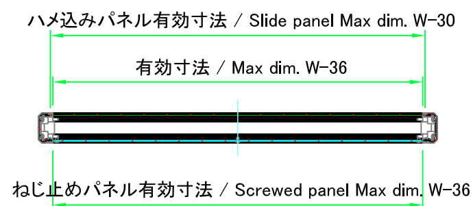
A-A ( 1 : 6.5 )
